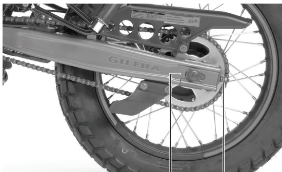
Eje de rueda trasera Tensor de cadena
