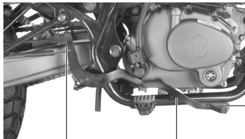
Tuerca de ajuste Pedal de freno 20~30mm
